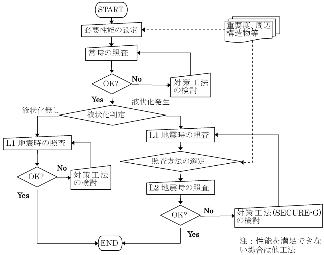
SECURE-G 工法の液状化時の変形照査適用フロー
